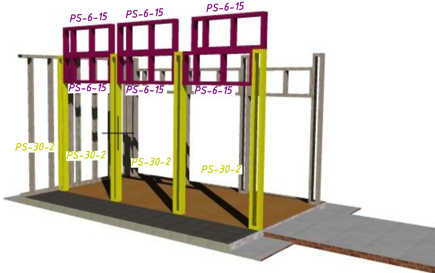
Типовые модульные панели из профиля
