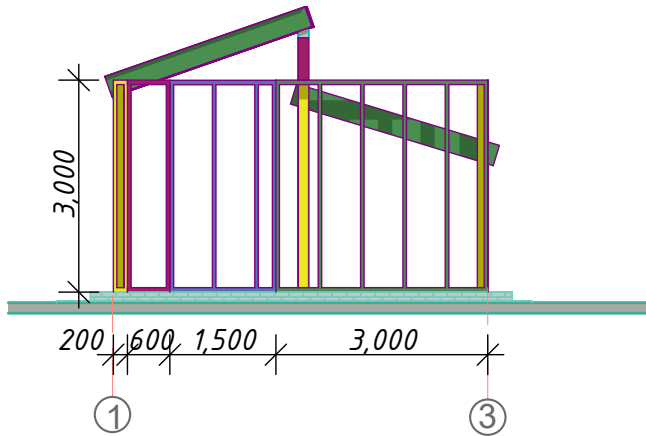
Фасад в осях 1-3
