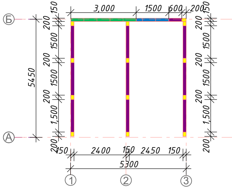
План расположения стеновых панелей
