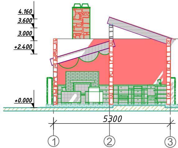
Фасад 1-3
