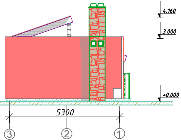
Фасад 3-1
