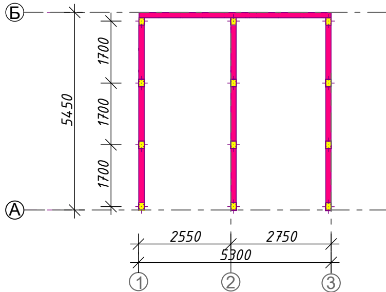
План беседки
