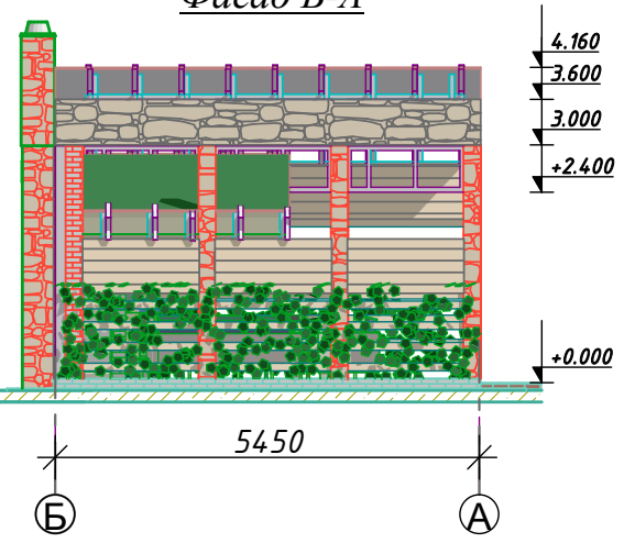
Фасад Б-А
