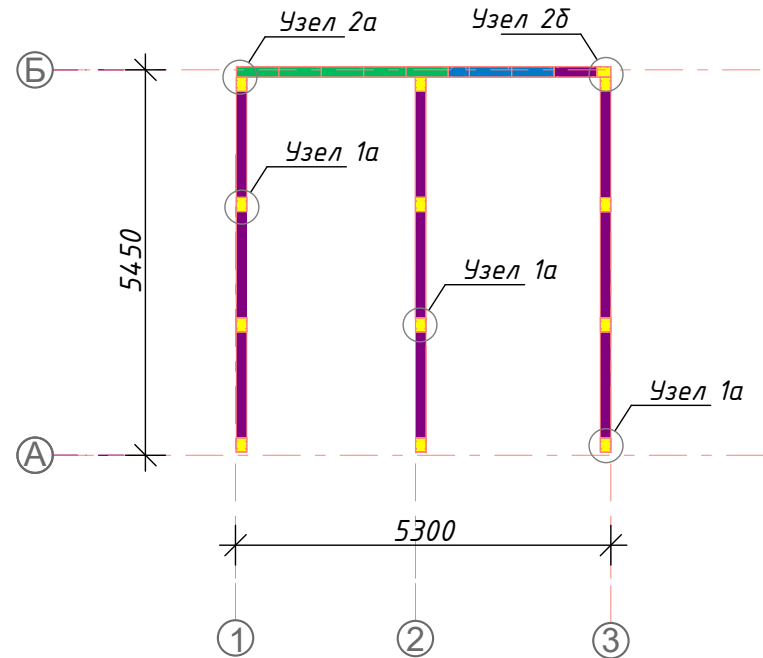
План расположения узлов
