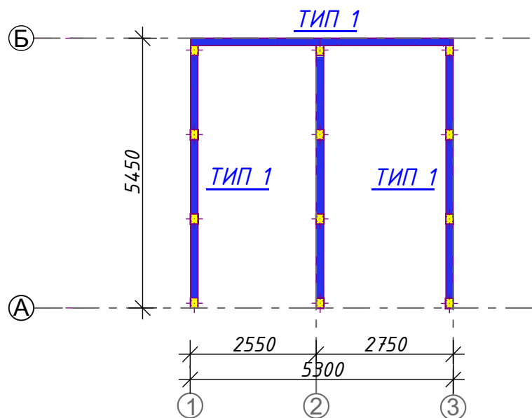
План расположения стеновых панелей
