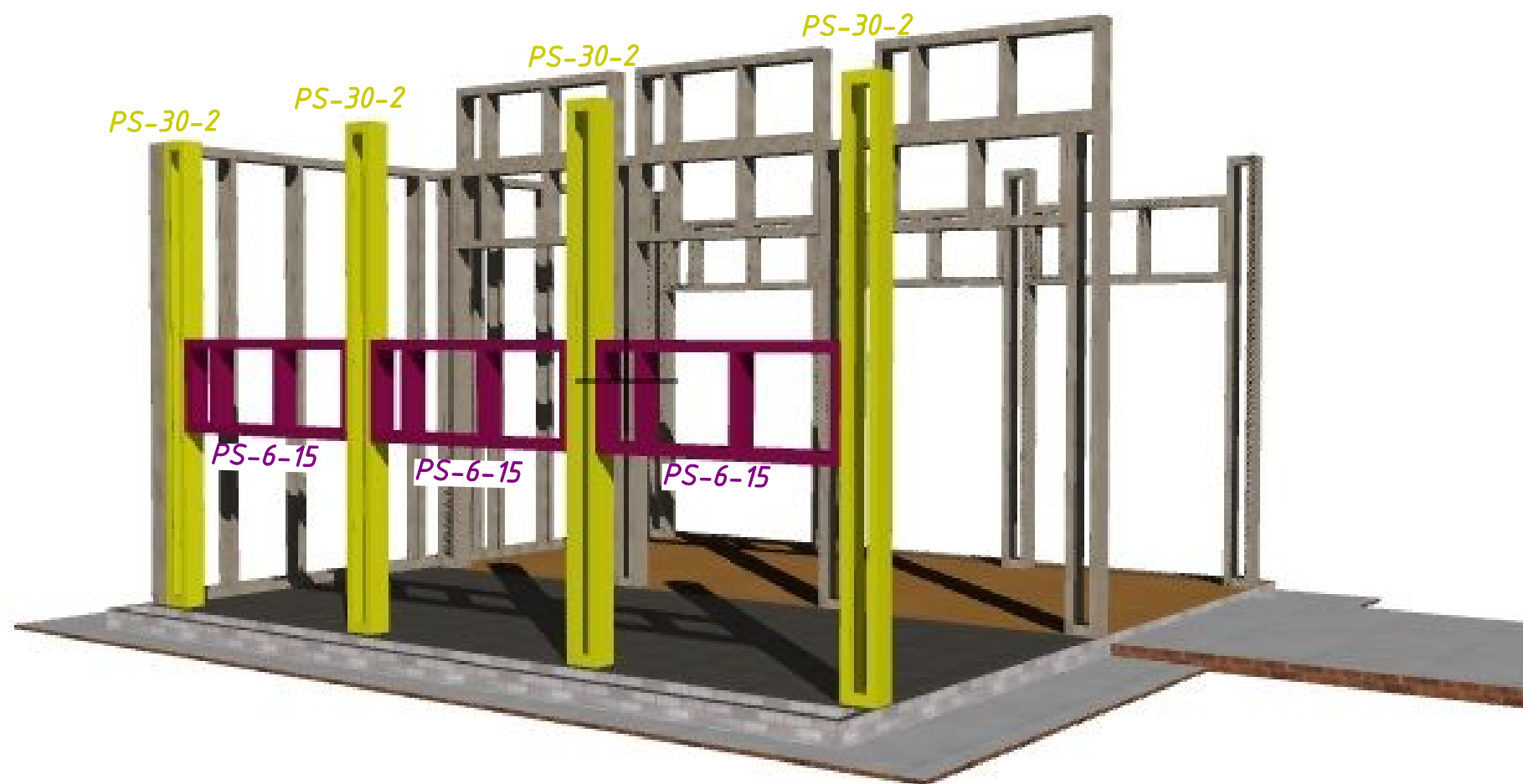
Типовые модульные панели из профиля
